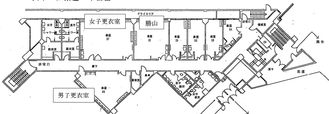
大ホール楽屋 平面図
