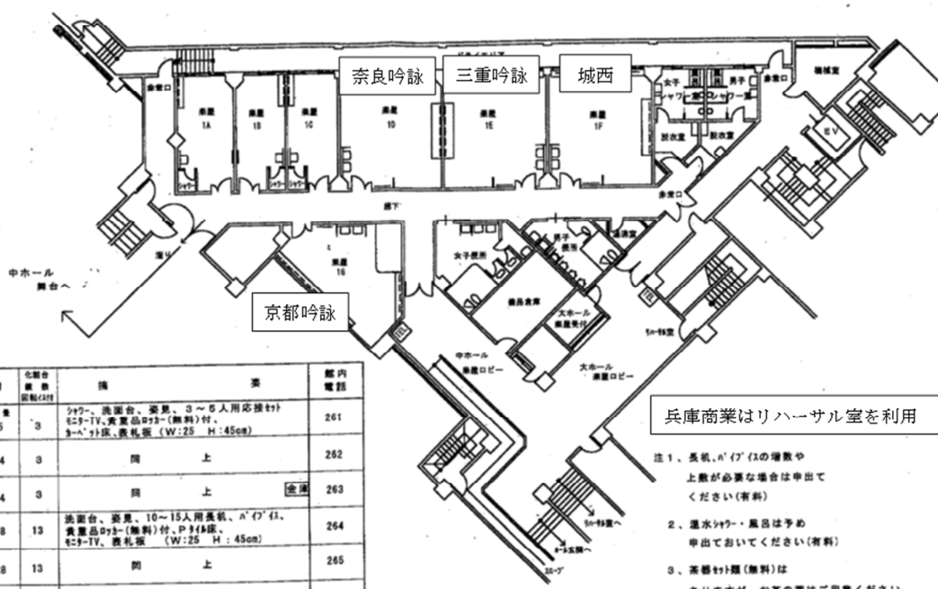
中ホール楽屋 平面図
